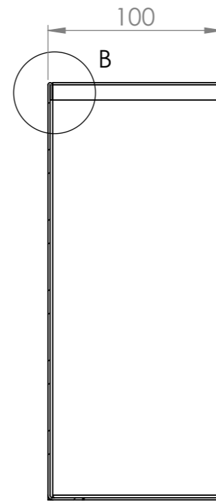
SECTION D-D
